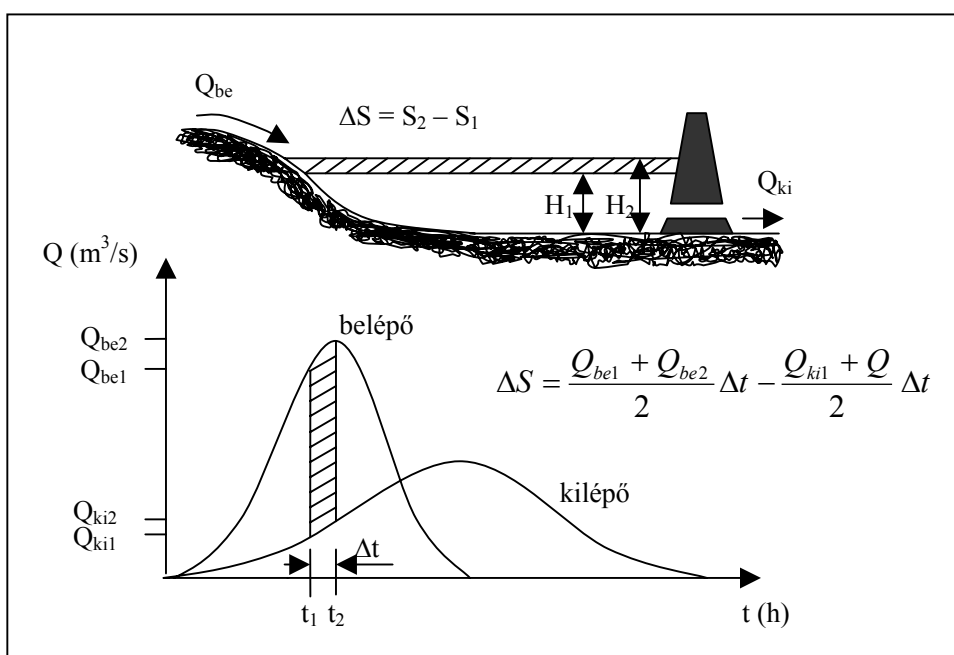
3.35 ábra. Záportározó elve
