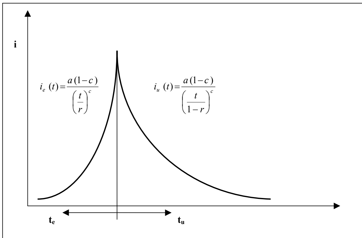
3.9 ábra. A Chicago tervezési csapadék
