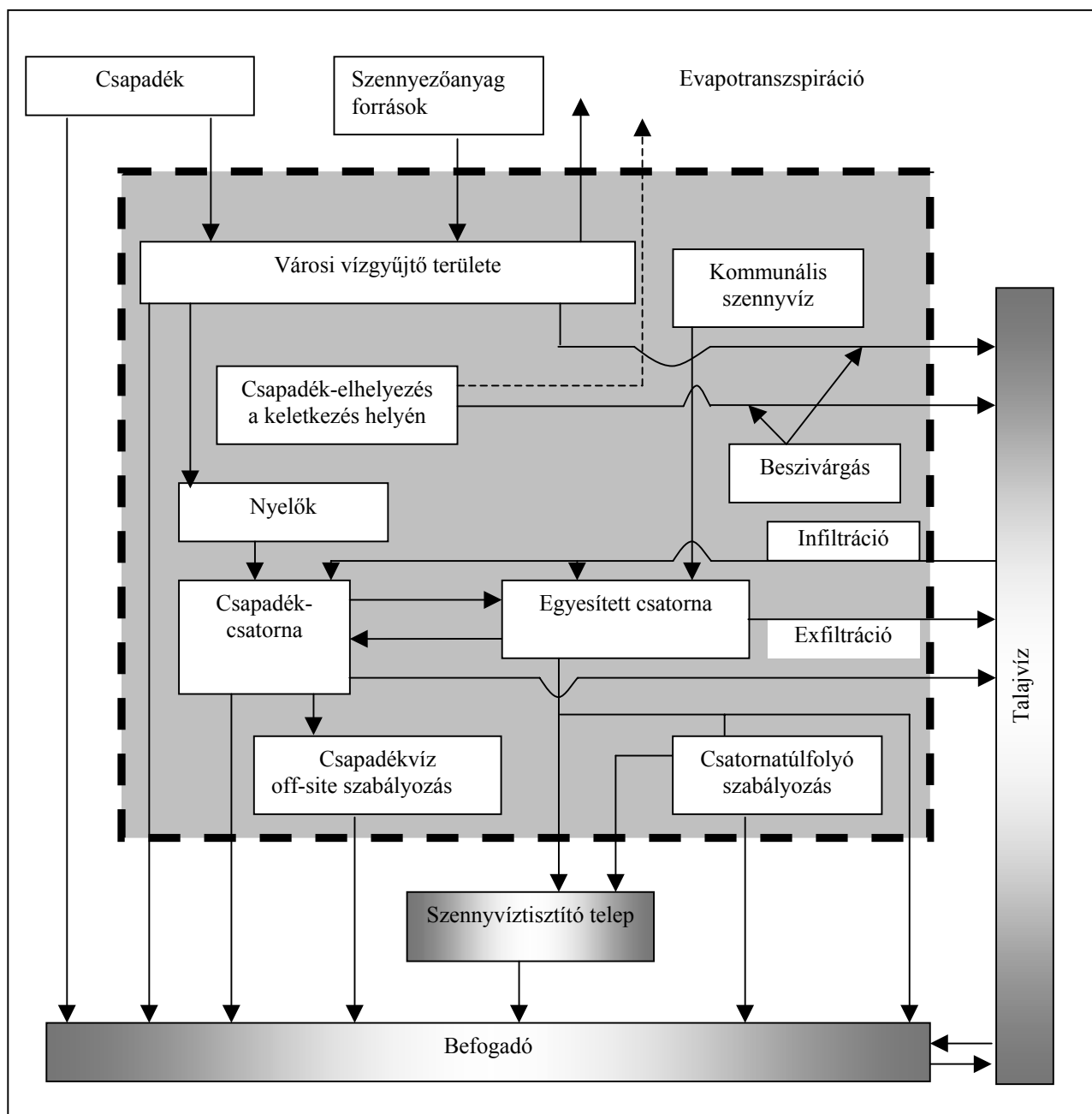
2.3 ábra. Az egyesített csatornahálózat elemei
