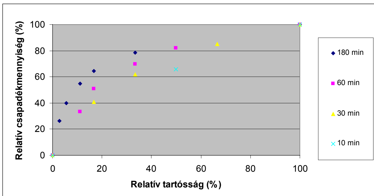
3.12 ábra. A rövididejű csapadékok magasságának aránya a tartósság relatív értékének függvényében
