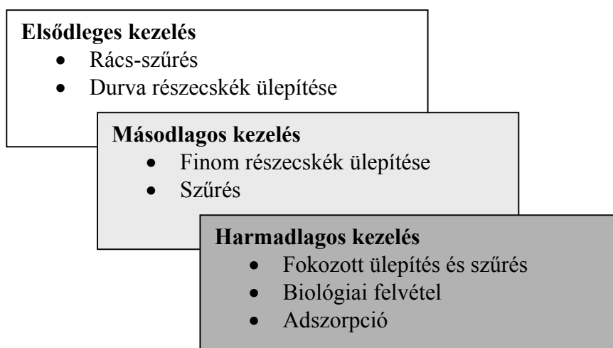
3.40 ábra. A csapadékvíz kezelés különböző szintjei
