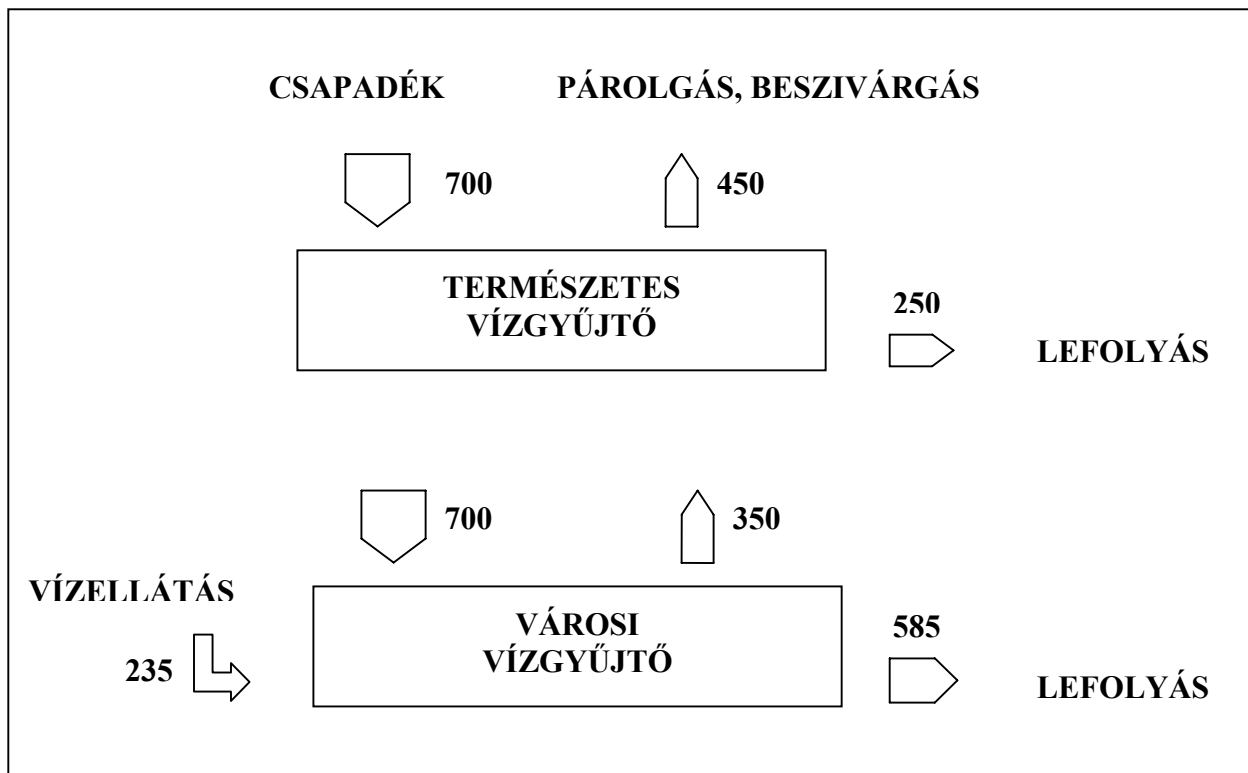
1.9 ábra. Sematikus vízmérleg természetes és városi vízgyűjtőn (mm)
