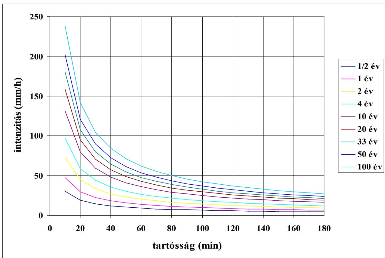
3.8 ábra. A magyar intenzitás–tartósság–gyakoriság (IDF) görbesor
