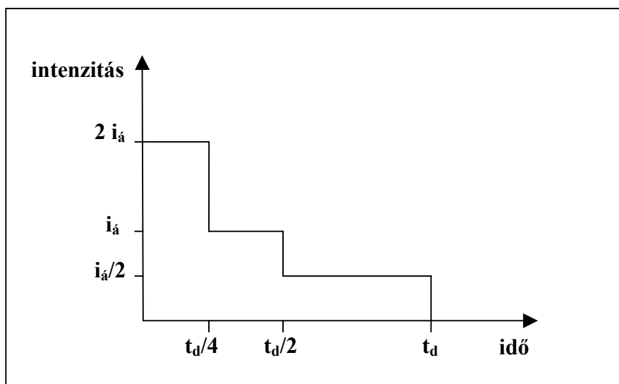
3.13 ábra. Kettős lépcsős alakú csapadékprofil
