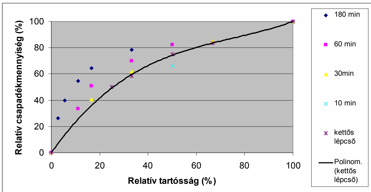
3.14 ábra. Mért csapadékok magasságának aránya a tartósság relatív értékének függvényében összehasonlítva a kettős lépcső alakú tervezési csapadék hasonló értékeivel
