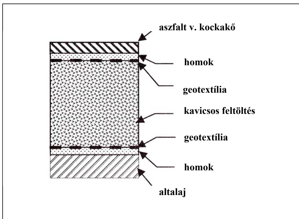
3.32 ábra. Porózus burkolat keresztmetszete (forrás: EPA NSW 1997)
