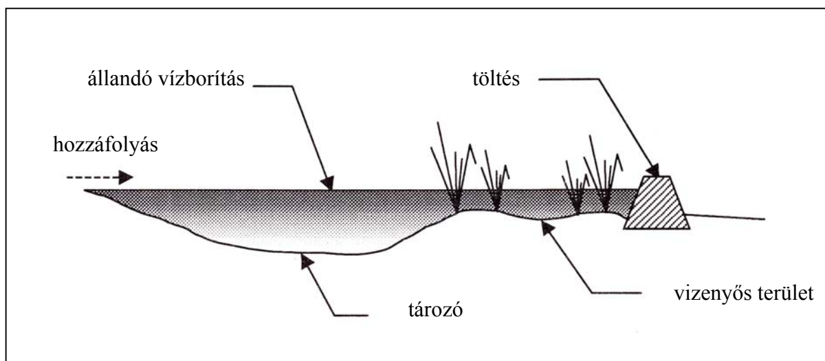
3.41 ábra. Gyökérzónás tisztítási rendszer (forrás: EPA NSW 1997)
