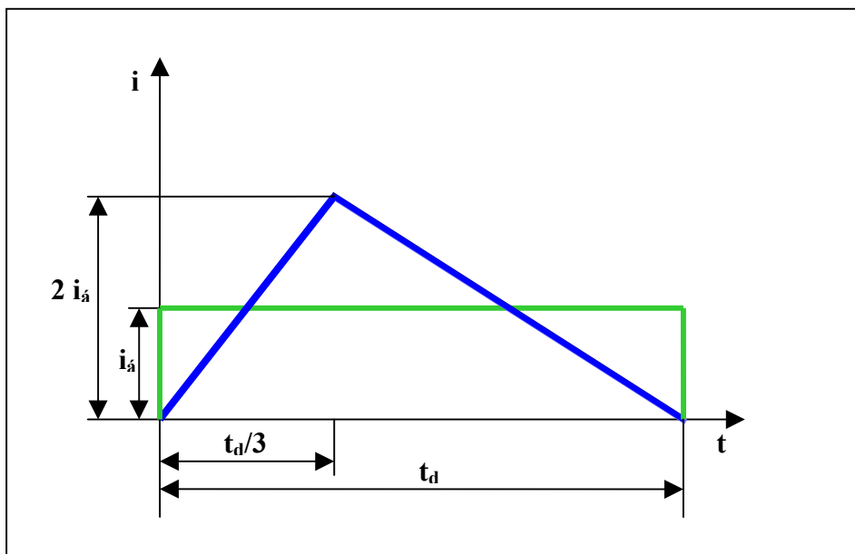
3.10 ábra. Háromszög alakú csapadék
