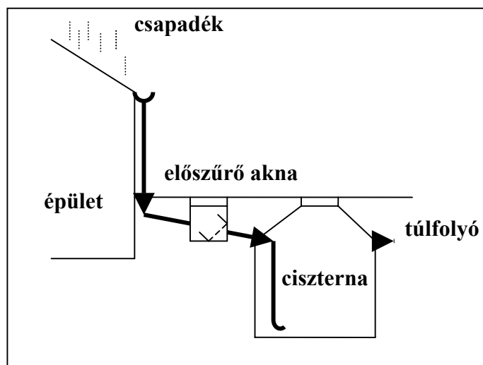
2.2 ábra. A tetővíz házi tározása
