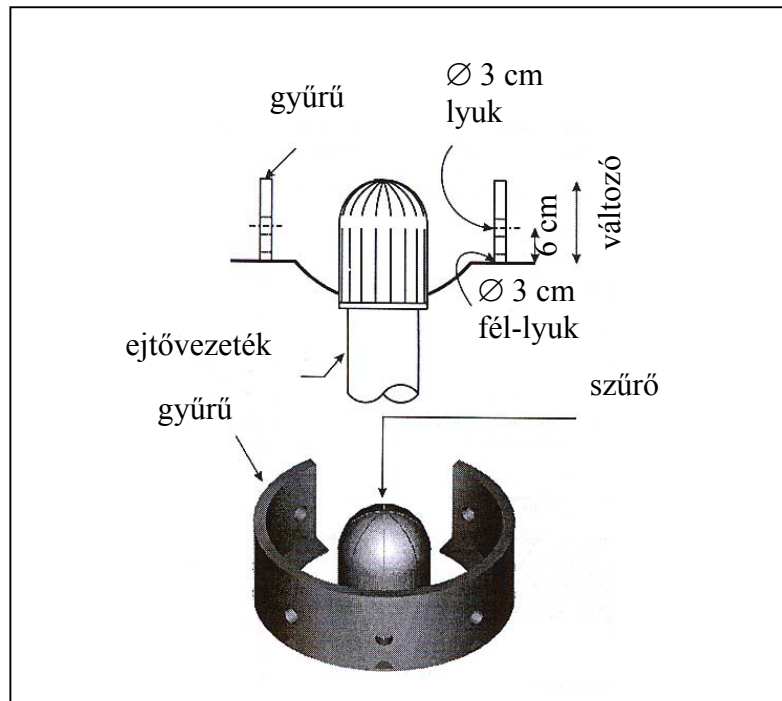
3.33 ábra. Tetőtározás érdekében használt szűrő
