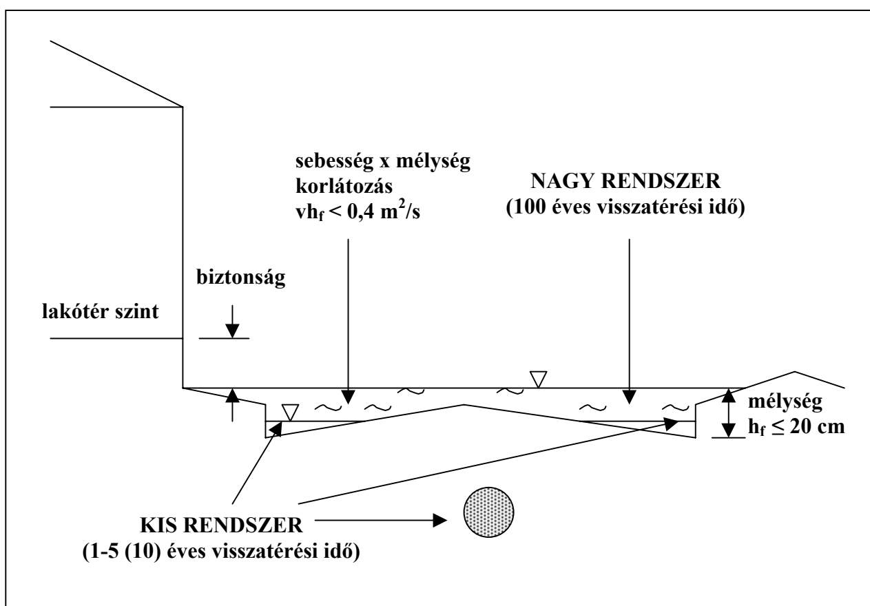
3.44 ábra. A kettős csatornázás koncepciója
