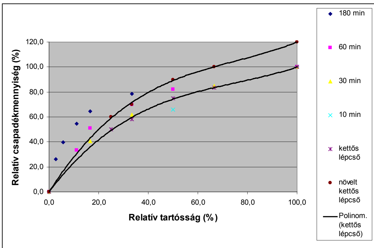
3.15 ábra Az egyszerű és a megnövelt kettős lépcső alakú tervezési csapadék összehasonlítása a mért csapadékokkal
