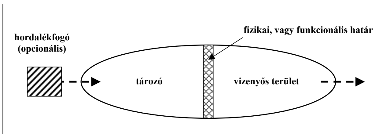
3.42 ábra. A gyökérzónás tisztítási rendszer funkcionális vázlata
