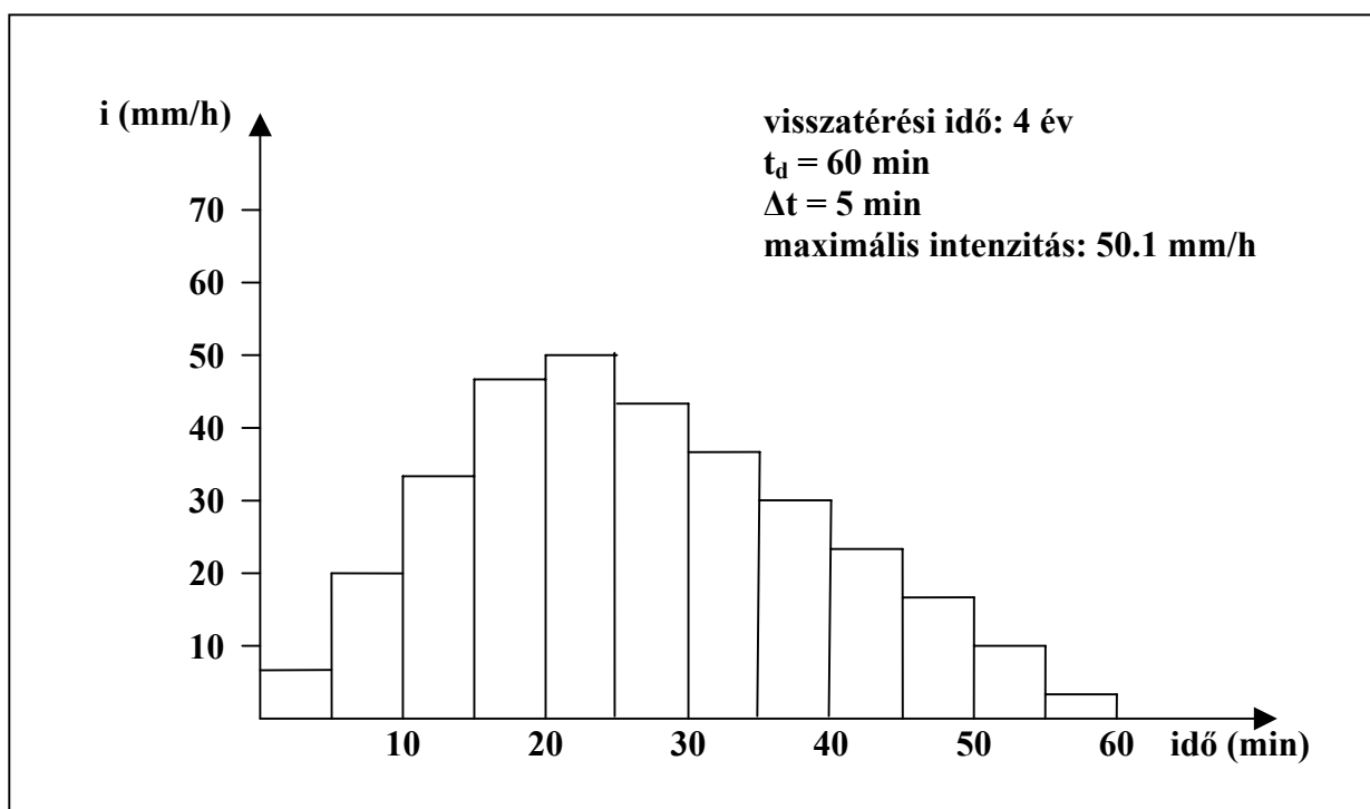
3.11 ábra. Háromszög alakú diszkrétizált csapadékinput a magyar csapadéktörvény alapján
