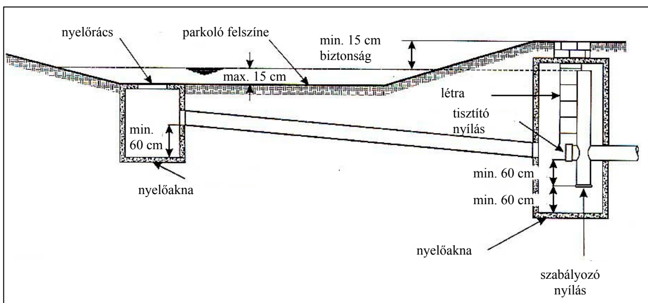
3.34 ábra. Tározás gépkocsi parkolóban
