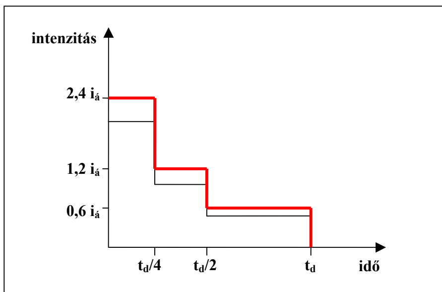
3.16 ábra Megnövelt kettős lépcső alakú tervezési csapadék
