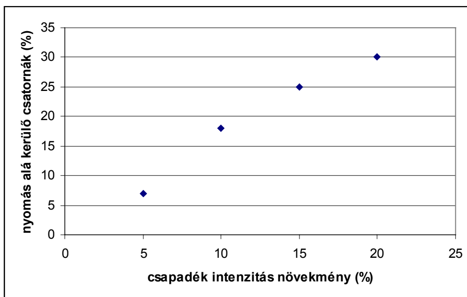
3.17 ábra. A csapadék intenzitásának függvényében nyomás alá kerülő csatornák aránya (forrás: Watt et al. 2003)
